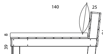
ZIJAAANZICHT
