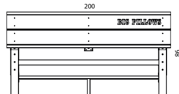
VOORAANZICHT
