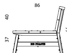
ZIAANZICHT
