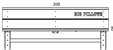
VOORAANZICHT
