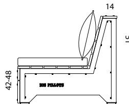
ZIJAAANZICHT
