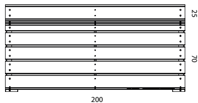
BOVENAANZICHT
