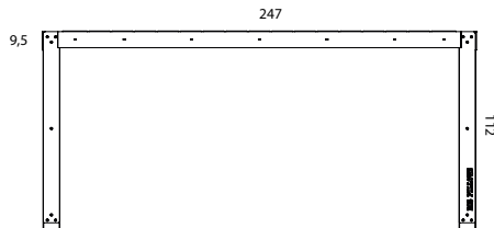
VOORAANZICHT
