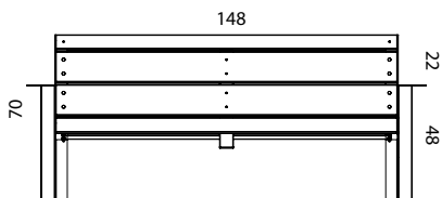
VOORAANZICHT
