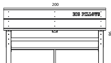
VOORAANZICHT
