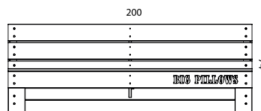
VOORAANZICHT
