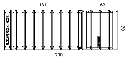
BOVENAANZICHT
