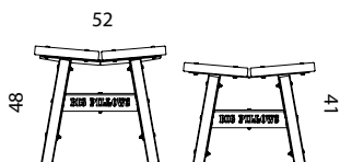
ZIJAANZICHT
