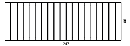
BOVENAANZICHT
