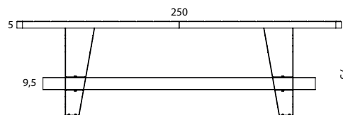
VOORAANZICHT
