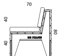
ZIJAAANZICHT
