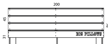
VOORAANZICHT
