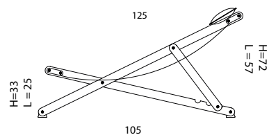
ZIJAAANZICHT
